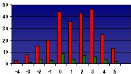
Raspodjela meteora po magnitudama
